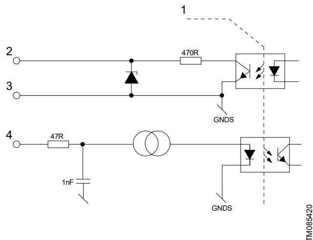
Skemaatiline joonis, samaväärne liides
