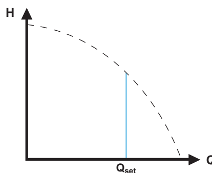
Ühtlase vooluhulga karakteristik
