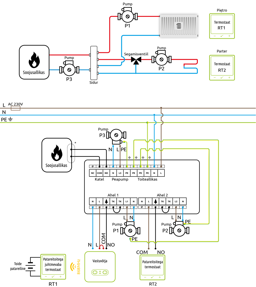
a) - Kahe küttesüsteemi ühendamine integraatoriga
