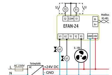
4-toruline ventilaator-konveieriga seade (kütmine ja jahutamine) - ventilaatori ja NC-tüüpi ajamite ühendamine
