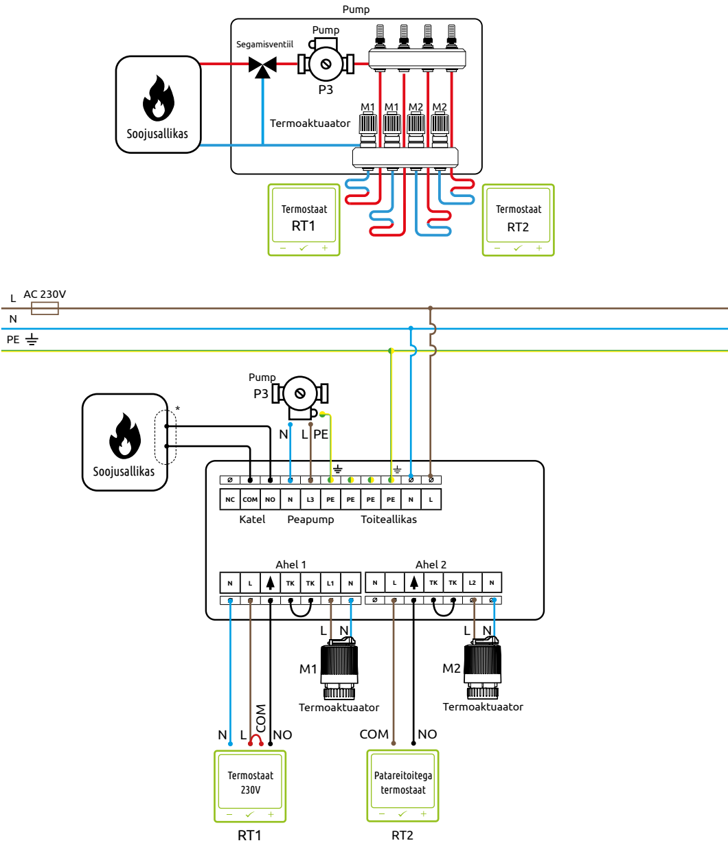
b) - Kahe pörandakütte tsooni ühendamine integraatoriga
