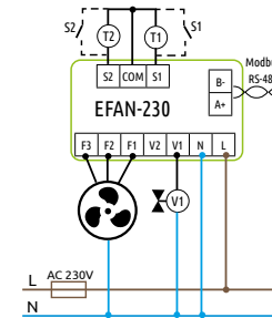
a) 2-toruline kliimakonvektor (kütmine ja/või jahutamine)
