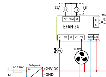
2-toruline kliimakonvektor (kütmine ja jahutamine) - ventilaatori ja NC-tüüpi täiturmehhanismi ühendamine
