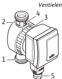
Ventielen
